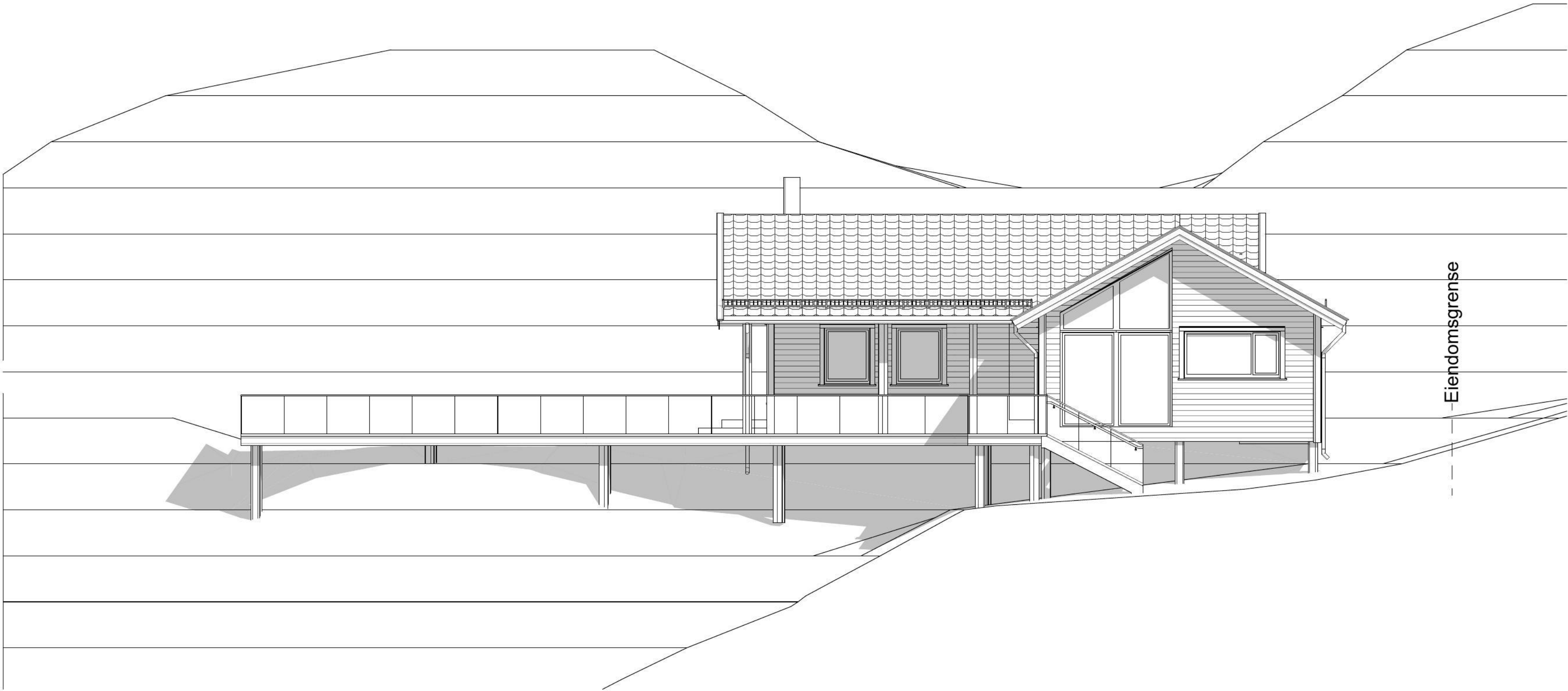
1:100 Fasade Vest
